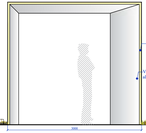
Pjūvis a-a:
