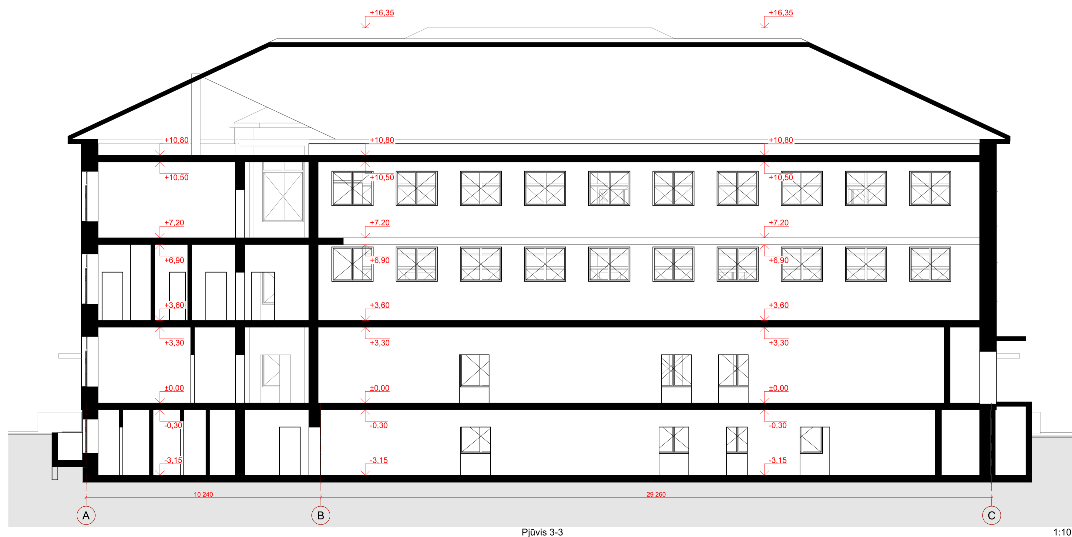
Pjūvis 3-3
