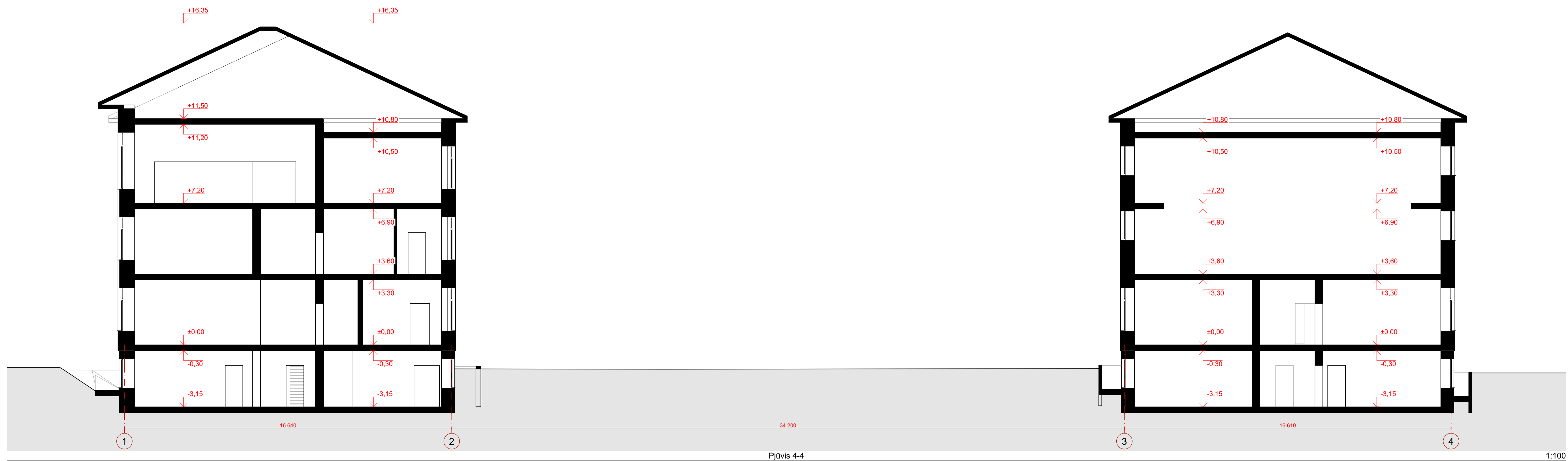
Pjūvis 4-4
